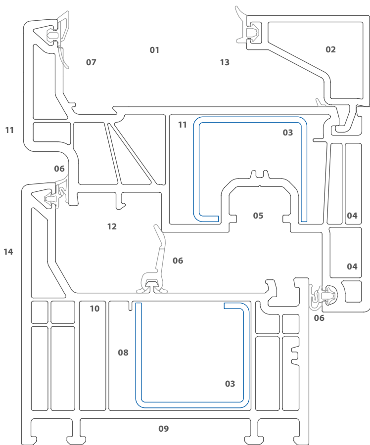
Elegante křídlo slícované s rámem v jedné rovině (obr. 1:1)
