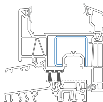
Elegantní práh balkonových dveří se zkosenou zasklívací lištou (obr. 1:2)
