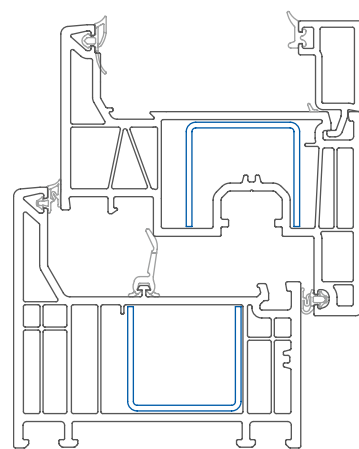
Elegante standardně odsazené křídlo (obr. 1:2)
