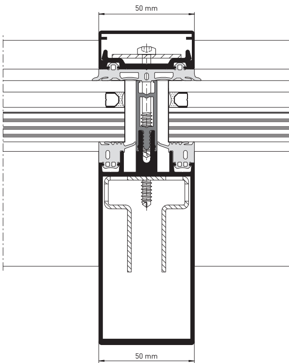
heroal C 50 FP, řez sloupkem v protipožární oblasti
