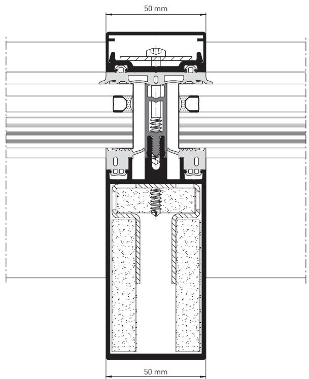
heroal C 50 FP, řez sloupkem v přechodové protipožární oblasti
