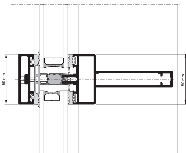
heroal C 50 ID, řez sloupkem s našroubovanou přítlačnou lištou (ocelová kontura)
