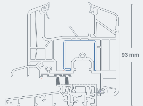
Novinka: Bezbariérový práh balkonových dveří Obr.: 1:2
