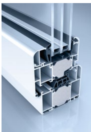
heroal W 72 RL – okenní systém se zaoblenou vnější konturou
